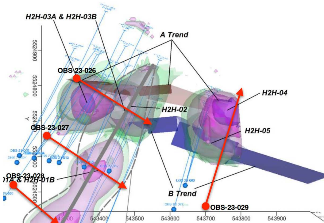
Figure 1 : programme de forage complété sur Obalski
